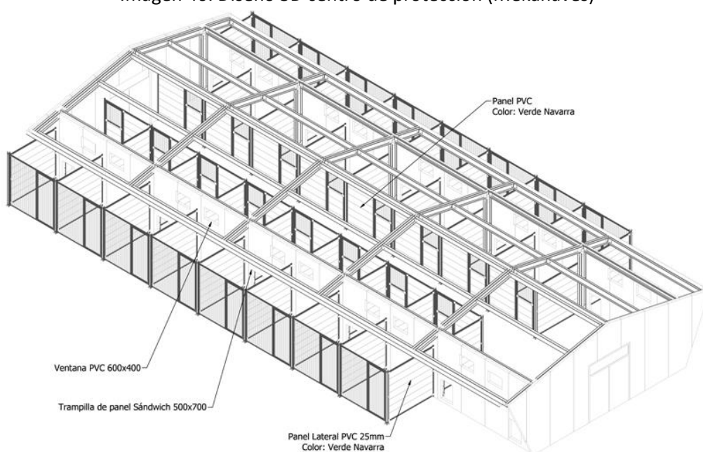
Imagen 40. Diseño 3D centro de protección (Mekanaves)
