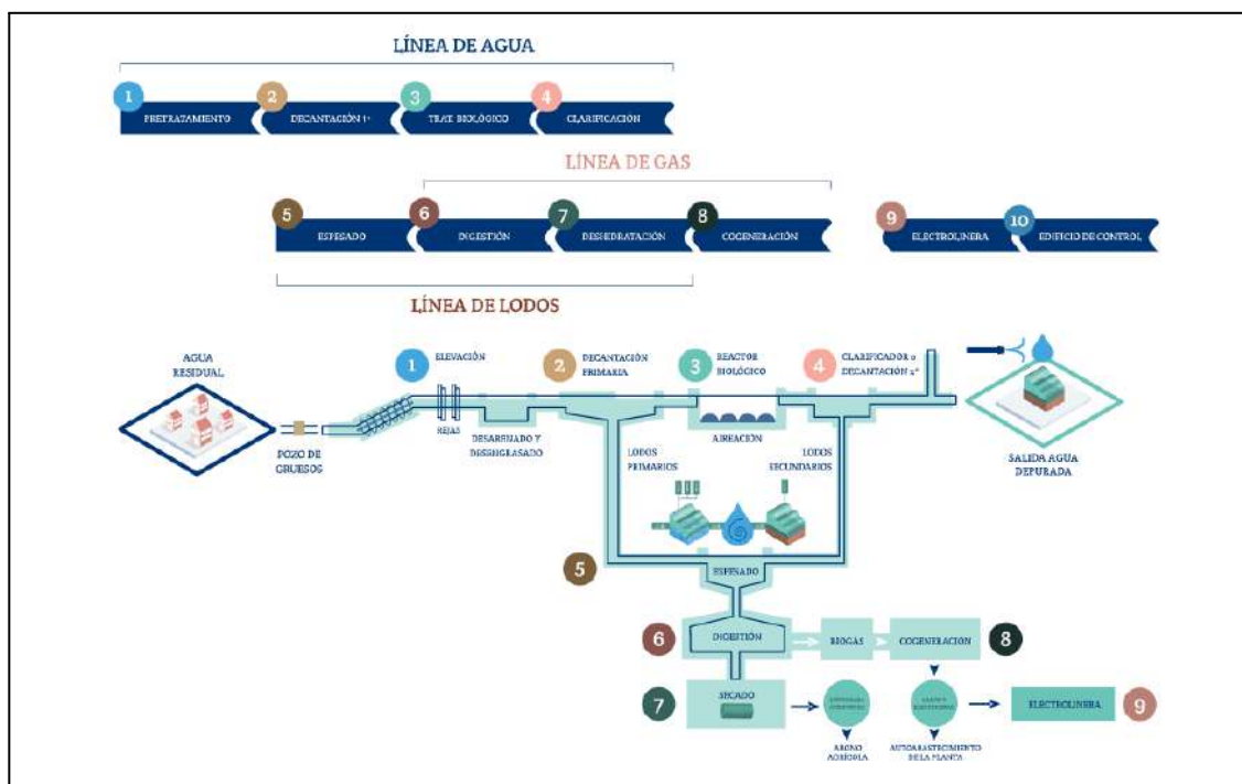
Imagen 17: Diagrama de proceso de la EDAR Sur de Emasagra. Fuente: EMASAGRA 2021, s. f.
