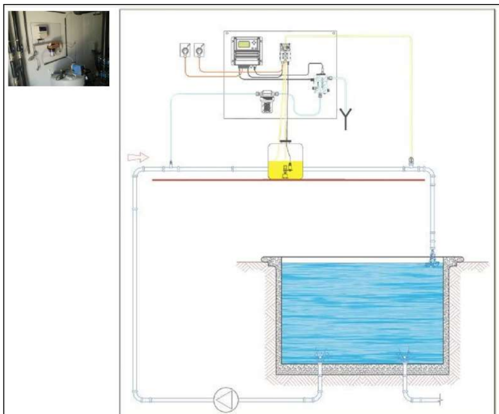
Imagen 26: Esquema de la cloración. Realizado por Ana Isabel Hernández Pérez de la empresa Hidrointec.
