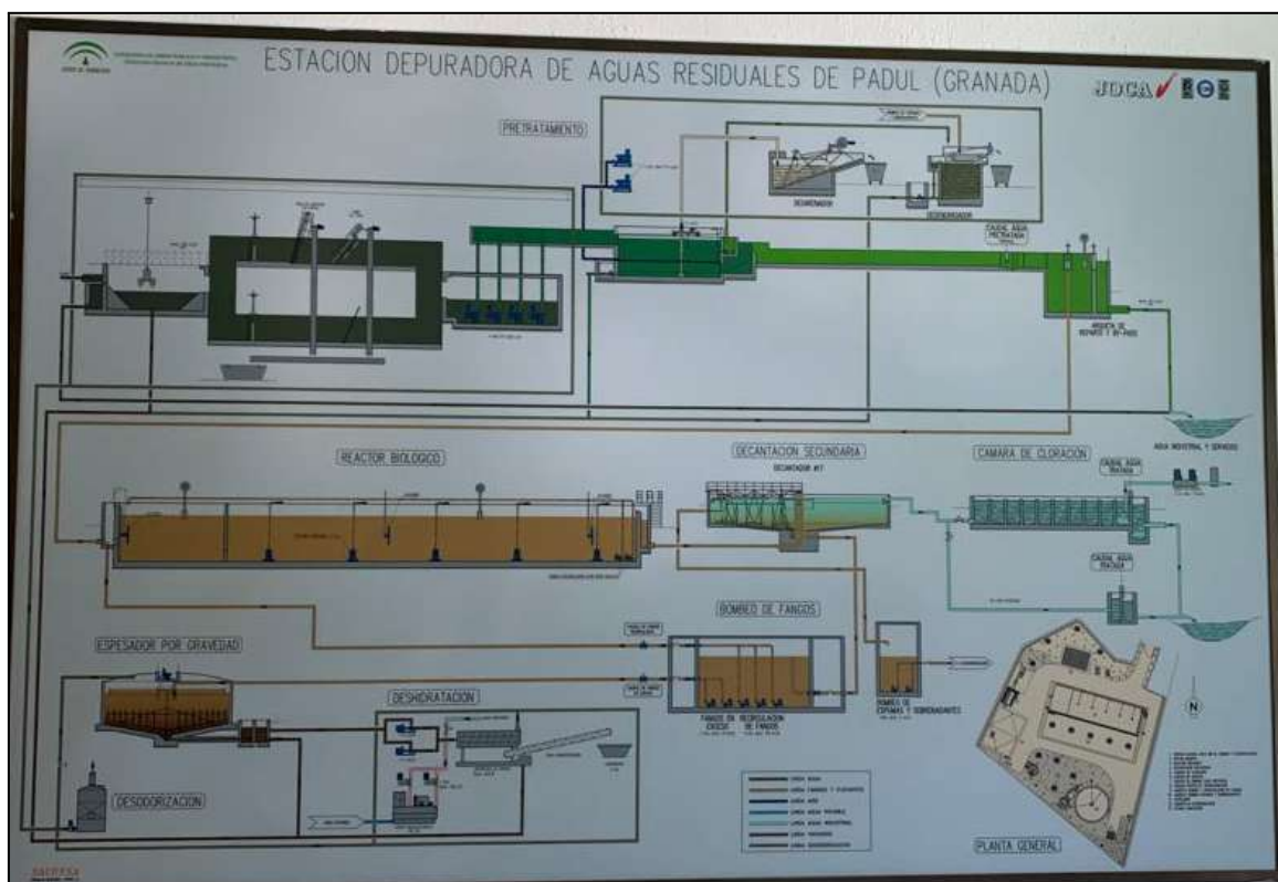
Imagen 11: Diagrama de la EDAR de Padul. Realizada por Almudena Sánchez
