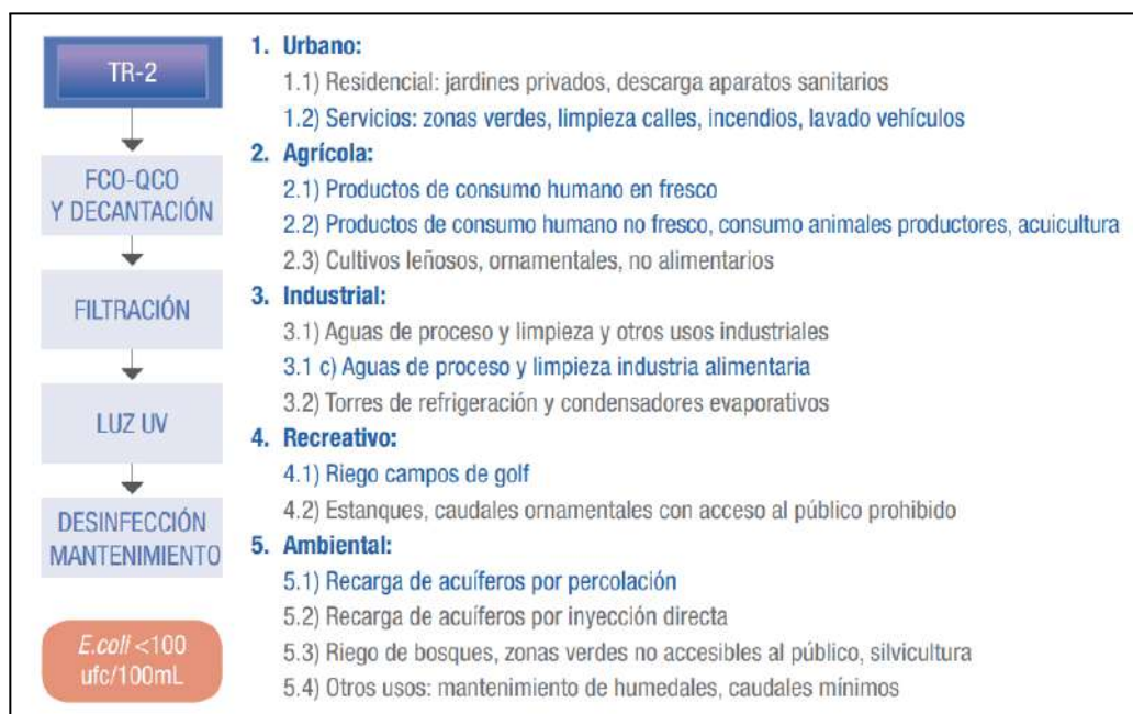
Imagen 21: Diagrama para el uso de recuperada para riego. Fuente: Reutilización de aguas depuradas , s. f.
