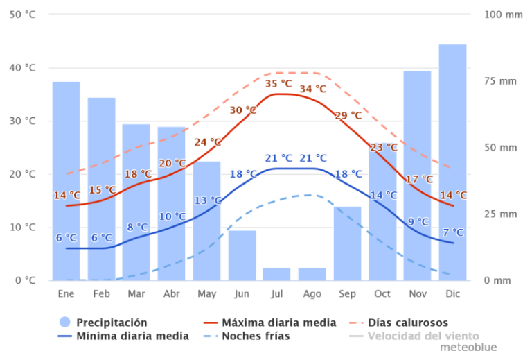
Ilustración 4: Climograma de Pinos Puente. Fuente: meteoblue
